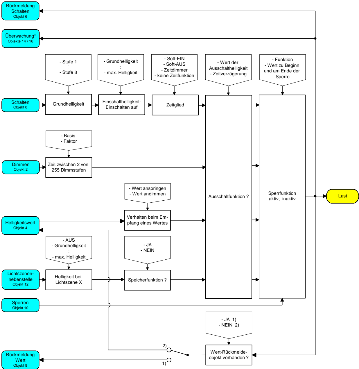
Funktionsschaltbild
