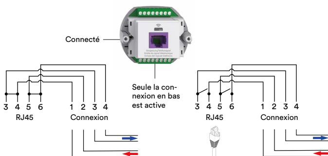
RJ45 non connectée
