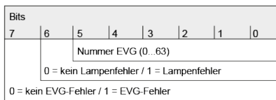
Bild 12: Telegrammaufbau 1-Byte-Fehlerstatus
