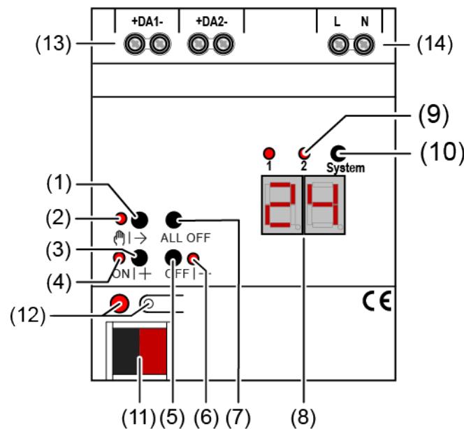
Bild 1: Geräteaufbau
