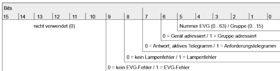
Bild 13: Telegrammaufbau 2-Byte-Fehlerstatus
