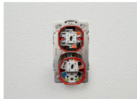
2. Anschliessend schnappen Sie die Apparate ein und fixieren diese.
